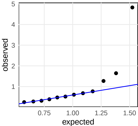
wachter qq-plot
